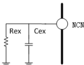
图 8-4 NCN 模式引脚的外接方式
